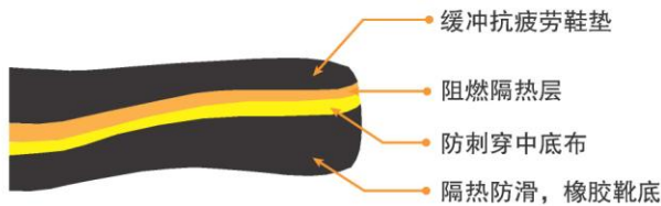
靴底分层结构
